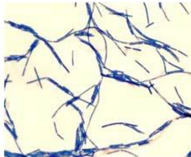
L.kefiranofaciens 菌株革兰氏染色的显微照片
