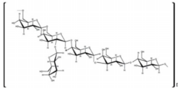
□开菲兰的一级结构
