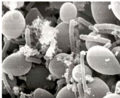
开菲尔颗粒表面的扫描电镜照片；酵母与杆菌共同存在
